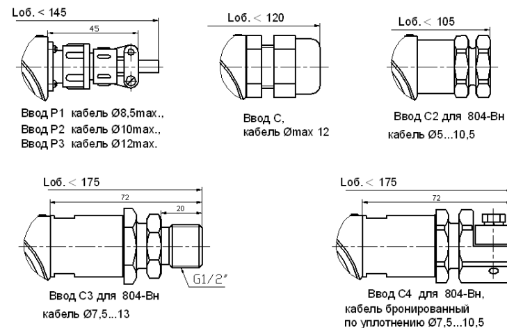
Вводы кабельные
