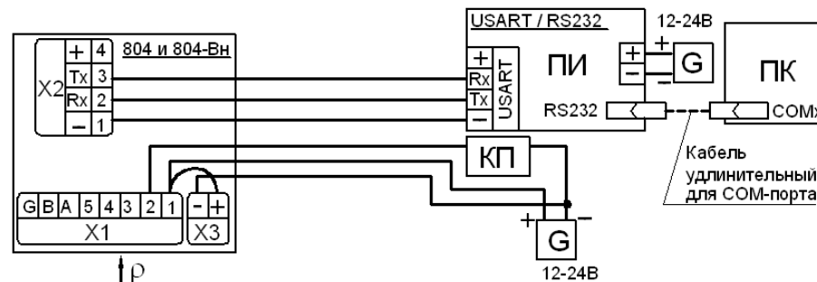
Рисунок В.7 - Схема подсоединения внешних электрических цепей плотномеров 804 и 804-Вн с выходными сигналами: цифровым USART и постоянным током 4-20мА (см. рис.В.2; ПИ – USART/RS232)
