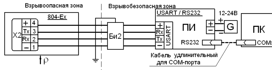
Рисунок В.11 - Схема подсоединения внешних электрических цепей плотномеров 804-Ех с цифровым выходным сигналом USART (см. рис.В.2 и В.9; ПИ – USART/RS232)
