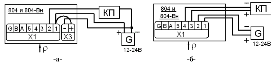
Рисунок В.6 - Схема подсоединения внешних электрических цепей плотномеров 804 и 804-Вн с выходным сигналом постоянного тока 4-20мА, -а- для газов и -б- для жидкостей
