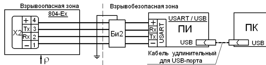
Рисунок В.12 - Схема подсоединения внешних электрических цепей плотномеров 804-Ех с цифровым выходным сигналом USART (см. рис.В.2 и В.9; ПИ – USART/USB)
