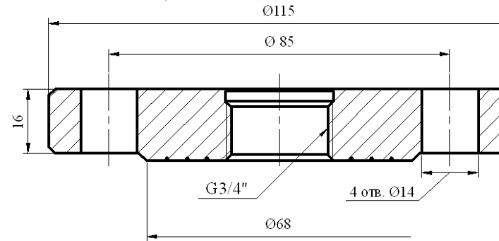
Рисунок А.6 - Бобышки монтажные
