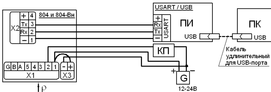
Рисунок В.8 - Схема подсоединения внешних электрических цепей плотномеров 804 и 804-Вн с выходными сигналами: цифровым USART и постоянного тока 4-20мА (см. рис.В.2; ПИ – USART/USB)
