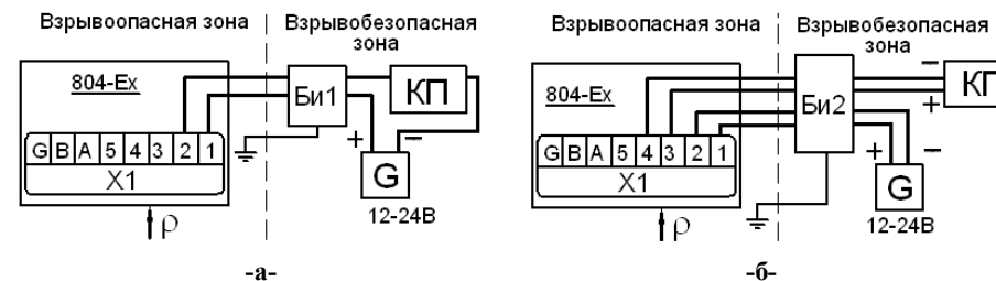
Рисунок В.13 - Схема подсоединения внешних электрических цепей плотномеров 804-Ех с выходным сигналом постоянного тока 4-20мА, -а- для газов и -б- для жидкостей
