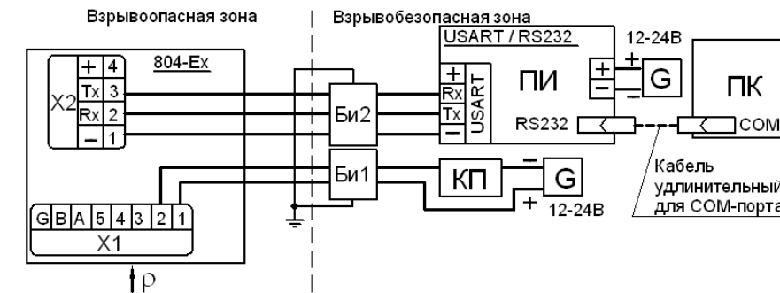
Рисунок В.14 - Схема подсоединения внешних электрических цепей плотномеров 804-Ех с выходными сигналами: цифровым USART и постоянного тока 4-20мА (см. рис.В.2 и В.9; ПИ – USART/RS232)
